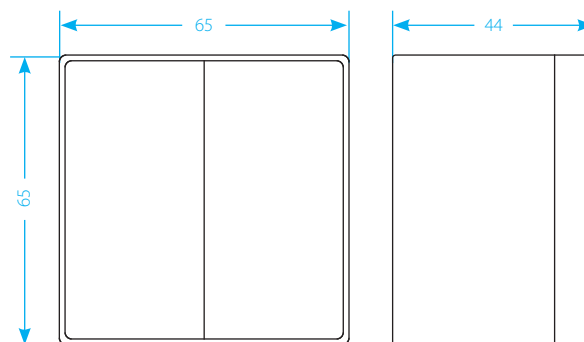
Выключатели IP44
