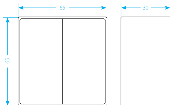
Выключатели IP20
