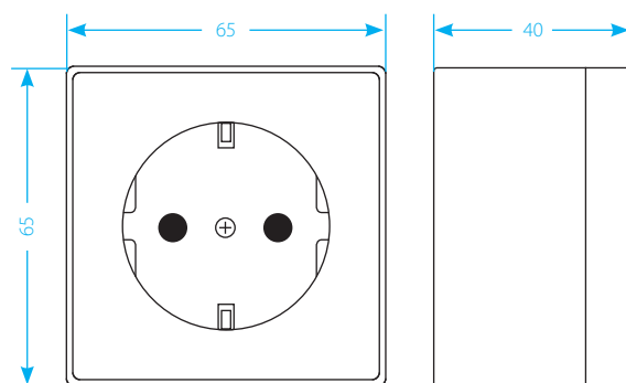
Розетка IP20
